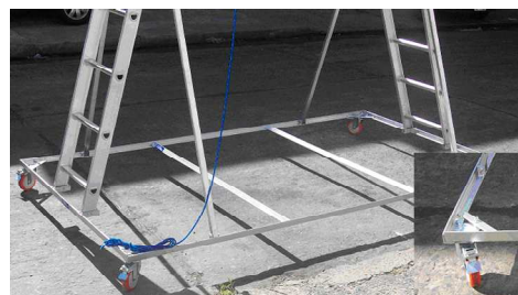
Base de Hierro con 4 Ruedas con freno
